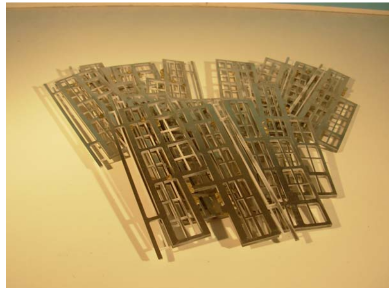
Weichentische vor der Lackierung (ca 120 Tische aus je 11 Einzelteilen)
